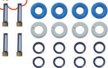
Conjunto c/4 filtros, 4 anéis, 4 discos de apoio e 8 anéis de vedação ASF0221
